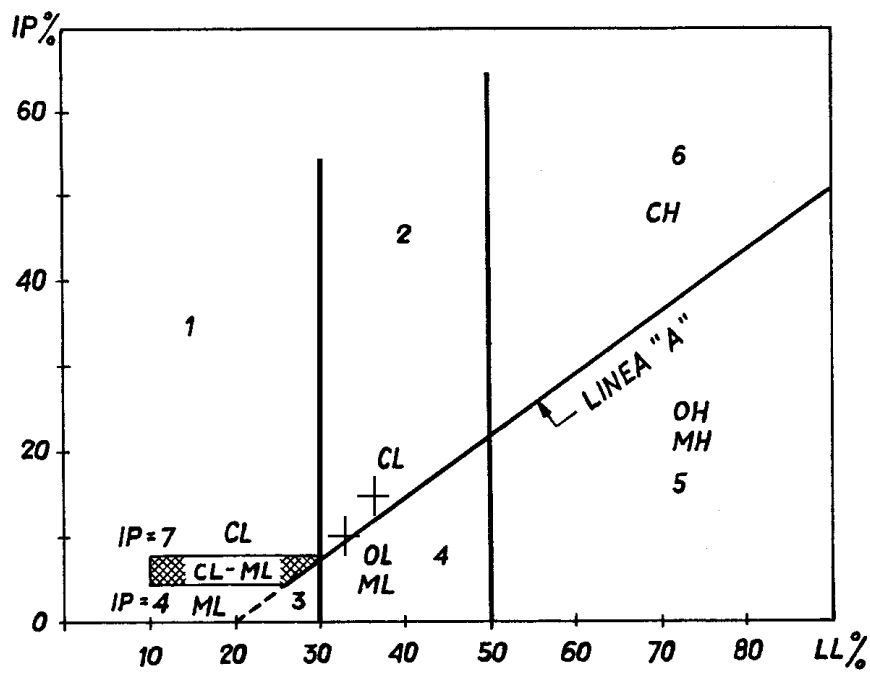
Carta di plasticità (*) (secondo A. Casagrande)
